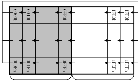
Display area 256dots Hidden area 256dots
