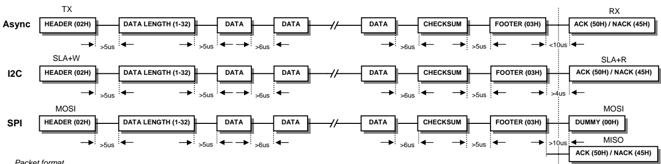
Packet format.
